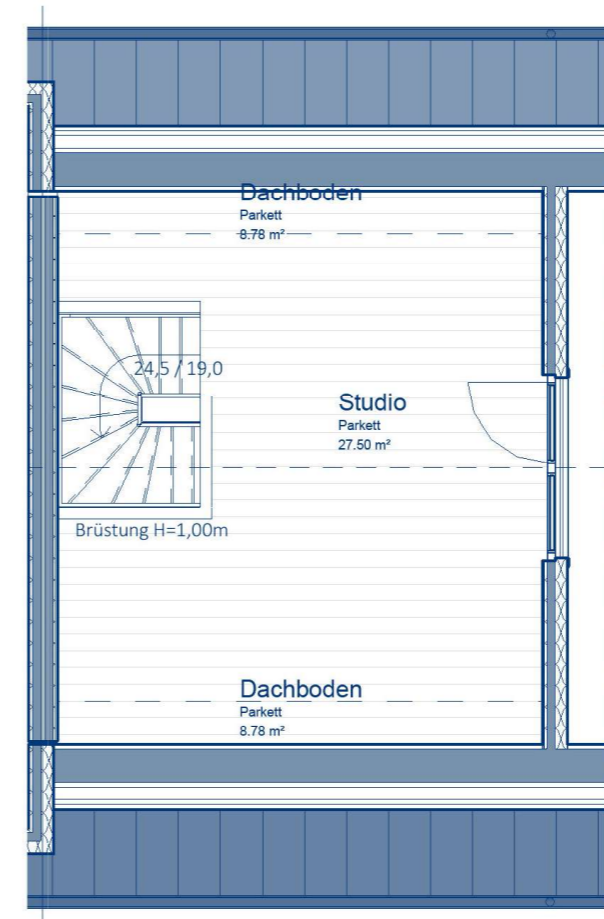
Dachgeschoß
