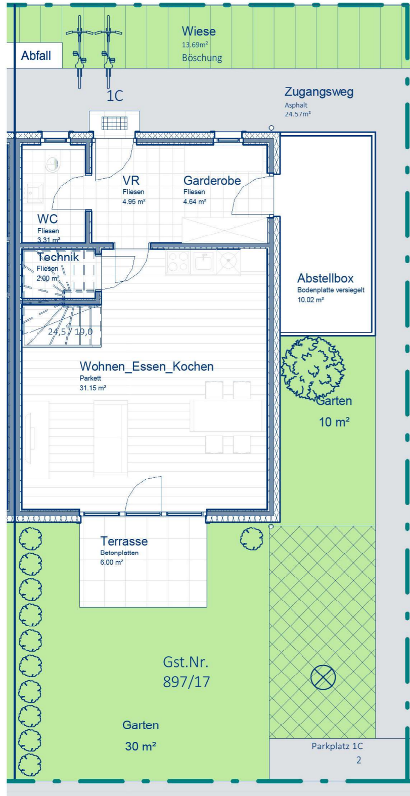
Erdgeschoß
