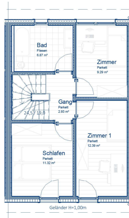
1. Obergeschoß
